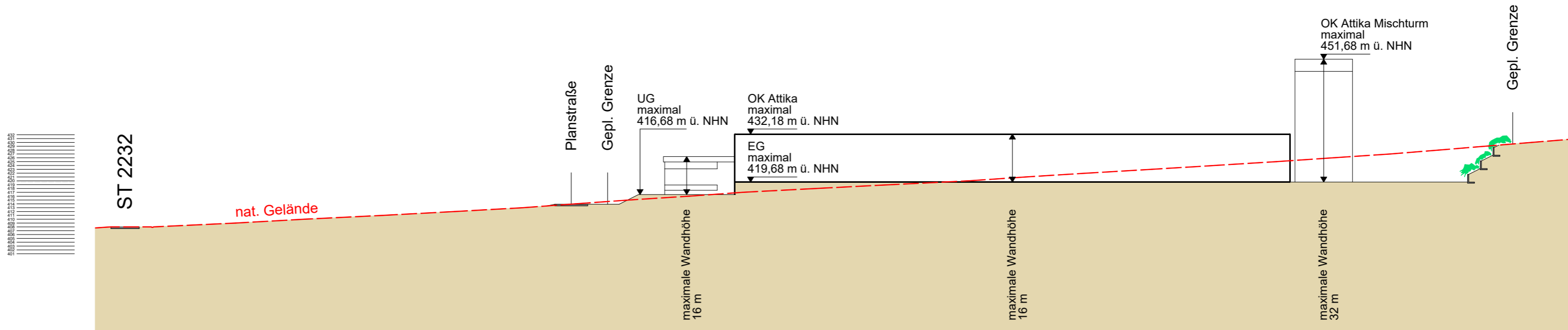
Schnitt D - D
